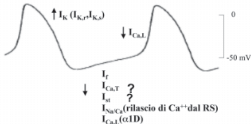
Rappresentazione di due PA delle cellule pacemaker del NSA. Correnti ioniche transmembrana e loro fase temporale di intervento nel meccanismo della depolarizzazione diastolica. La freccia ↓ indica correnti in ingresso (depolarizzanti), la freccia ↑ indica correnti in uscita (ripolarizzanti). La depolarizzazione del PM necessita della disattivazione delle correnti in uscita e dell'attivazione delle correnti in ingresso. Il punto interrogativo indica l'incertezza sul ruolo svolto (si veda il testo per le abbreviazioni). (Modificata da Kodama I. 8 )
