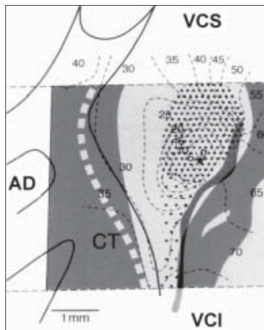
Rappresentazione schematica del NSA in sezione longitudinale (da preparazione di coniglio). In grigio chiaro: NSA; in grigio scuro: il tessuto atriale; tratteggio largo chiaro: zona del NSA sovrapposta al muscolo atriale della crista terminalis; punteggiatura: strati di cellule del NSA; stella: pacemaker principale del NSA. Isocrone, con tempo (in ms) di propagazione del potenziale d’azione dal pacemaker principale alle varie zone del NSA e dell’atrio indicate dalle linee tratteggiate. VCS, vena cava superiore; VCI, vena cava inferiore; AD, atrio destro; CT, crista terminalis. (Modificata da Boyett MR. 4 )
